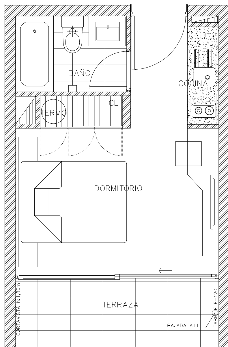
PLANTA DE ESTUDIO 203 AL 803
