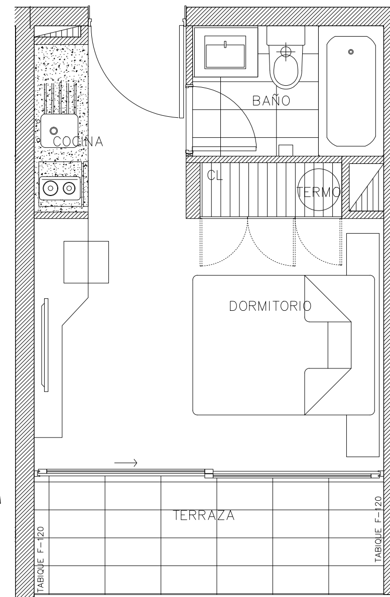
PLANTA DE ESTUDIO 204 AL 804
