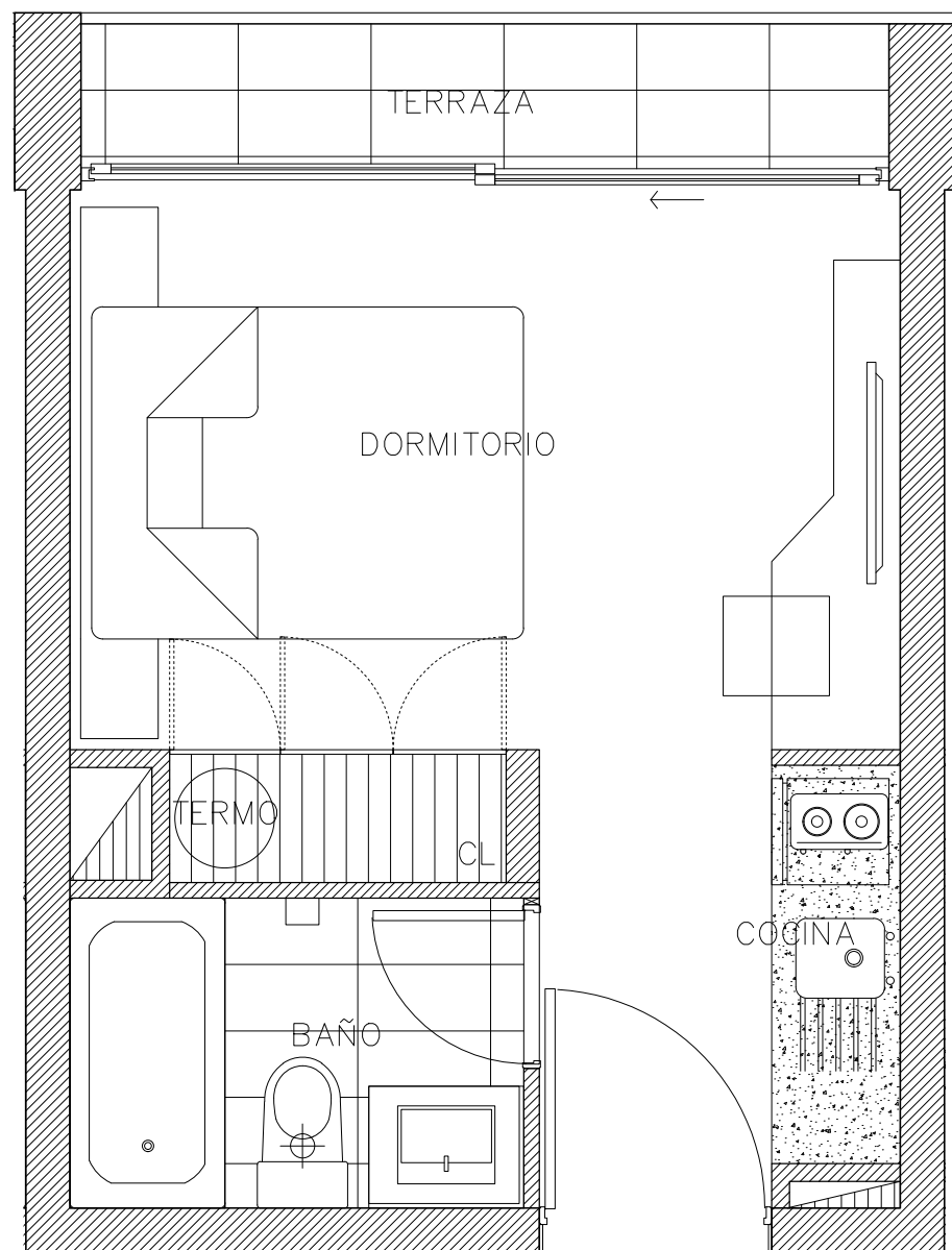
PLANTA DE ESTUDIO 209 AL 809
