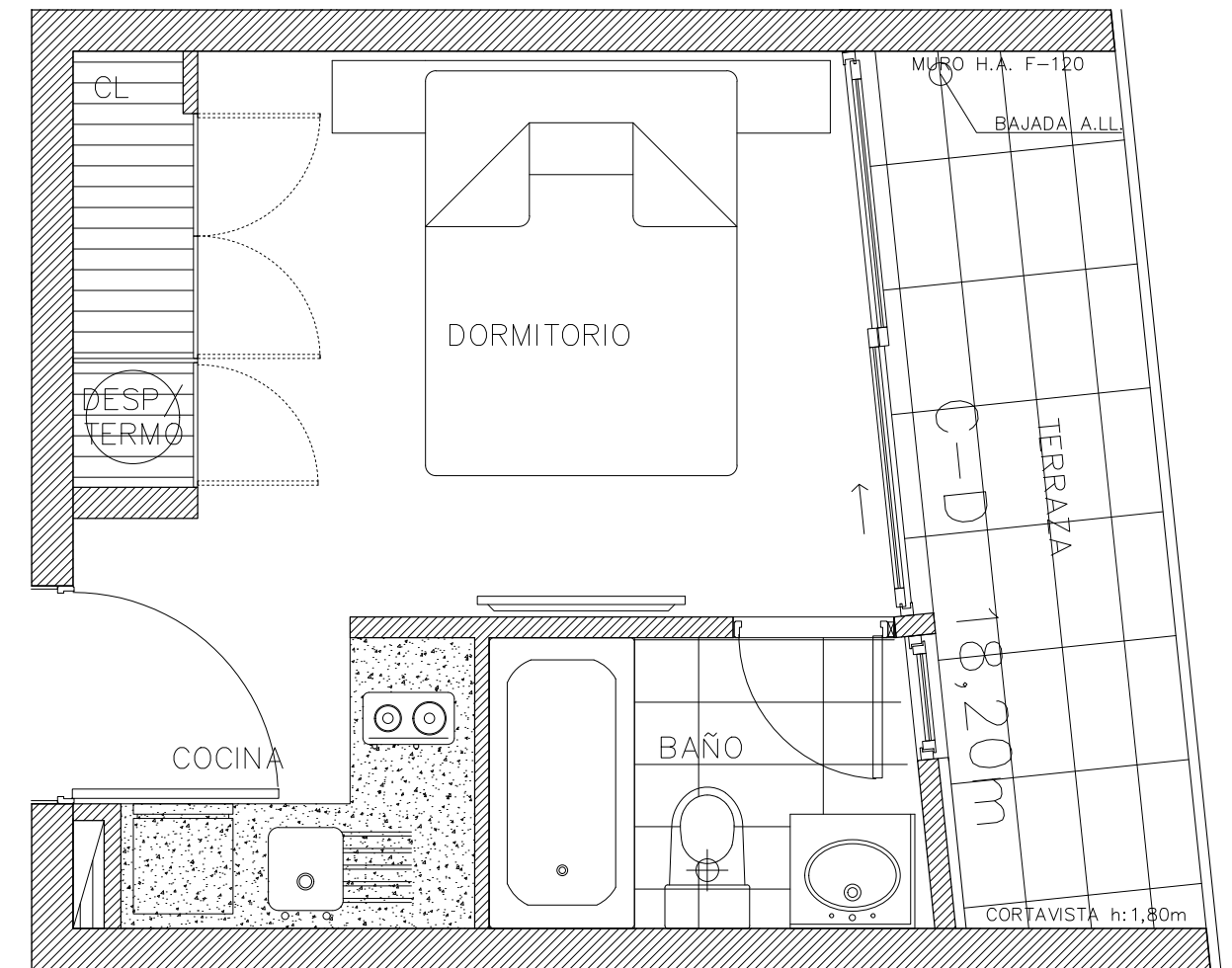
PLANTA DE ESTUDIO 314 AL 814
