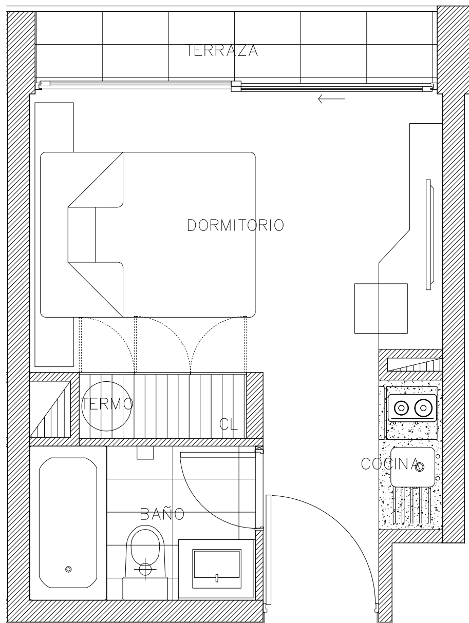
PLANTA DE ESTUDIO 211 AL 811
