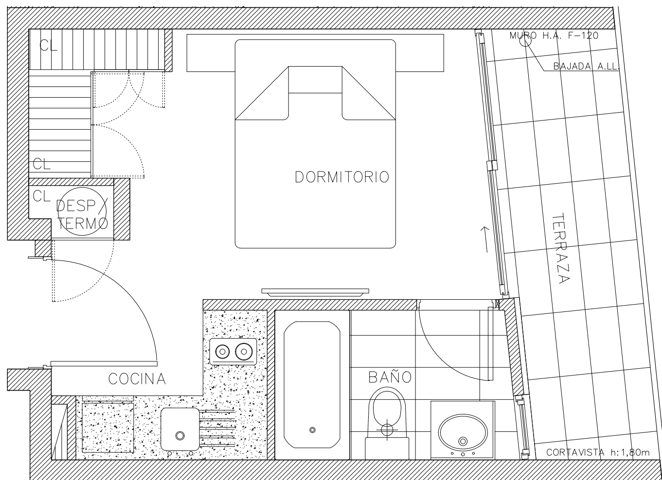
PLANTA DE ESTUDIO 315 AL 815
