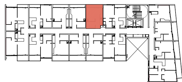
PLANTA DE ESTUDIO 211 AL 811
